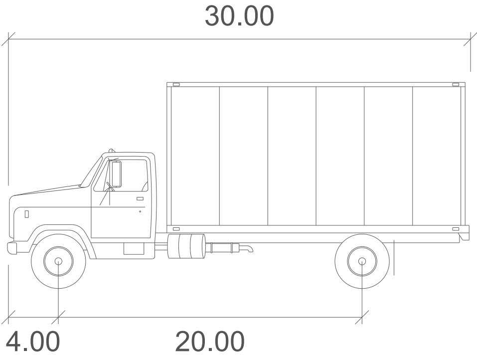
SU-30
